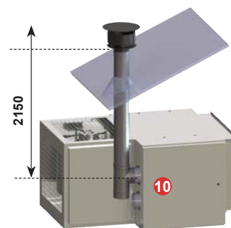
Вертикальный дымоход B22 Максим. длина 8м
