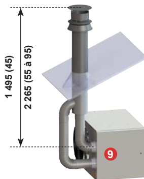
Вертикальный коксиальный дымоход C32 Максим. длина 8м
