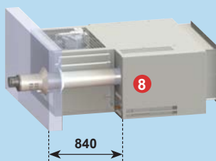
Горизонтальный коаксиальный дымоход C12 Максим. длина 6м
