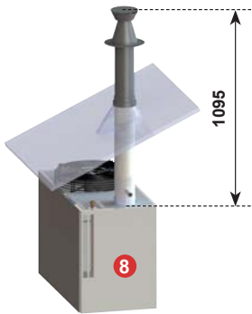
Вертикальный коксиальный дымоход C32 Максим. длина 6м
