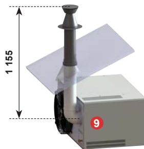
Вертикальный коксиальный дымоход C32 Максим. длина 6м
