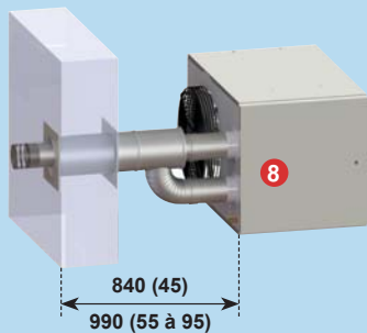
Горизонтальный коксиальный дымоход C12 Максим. длина 6м
