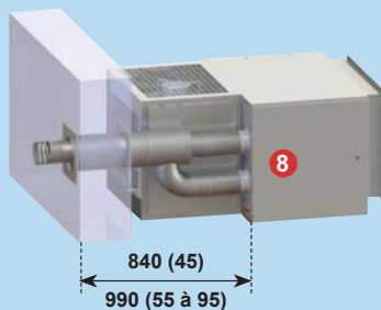
Горизонтальный коаксиальный дымоход C12 Максим. длина 6м
