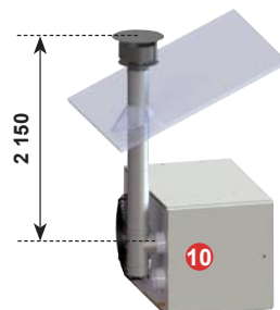
Вертикальный дымоход B22 Максим. длина 8м
