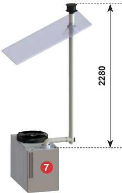
Вертикальный дымоход B22 Максим. длина 8м
