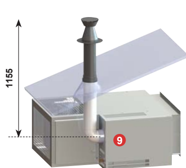
Вертикальный коаксиальный дымоход C32 Максим. длина 6м
