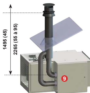
Вертикальный коаксиальный дымоход C32 Максим. длина 8м
