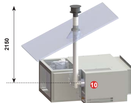
Вертикальный дымоход B22 Максим. длина 8м
