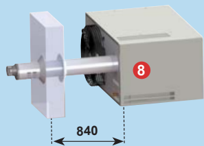
Горизонтальный коксиальный дымоход C12 Максим. длина 6м
